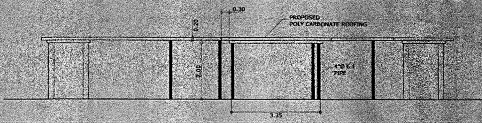
FRONT ELEVATION SCALE: 1:50
