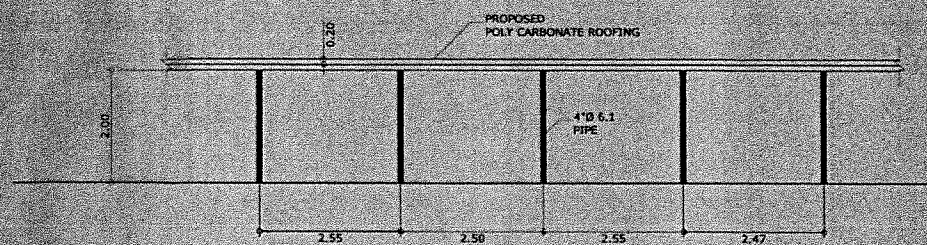
SIDE ELEVATION SCALE: 1:50
